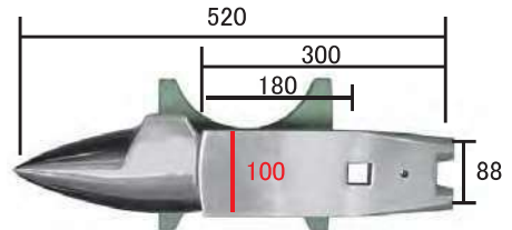
No.700585 : ダイヤモンド スタダード 35kg ベース W250xD220xH225 □26Φ8
