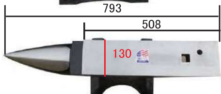
No.700590 : JHM Competitor 118kg ベース W310xD280xH340 □30Φ18
