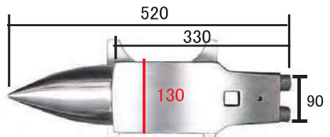
No.700586 : ダイヤモンド ラージ 38kg ベース W250xD220xH225 □26Φ9
